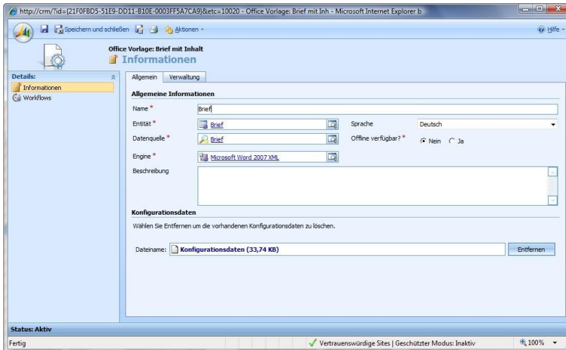
Abbildung 2 Vorlagenverwaltung
