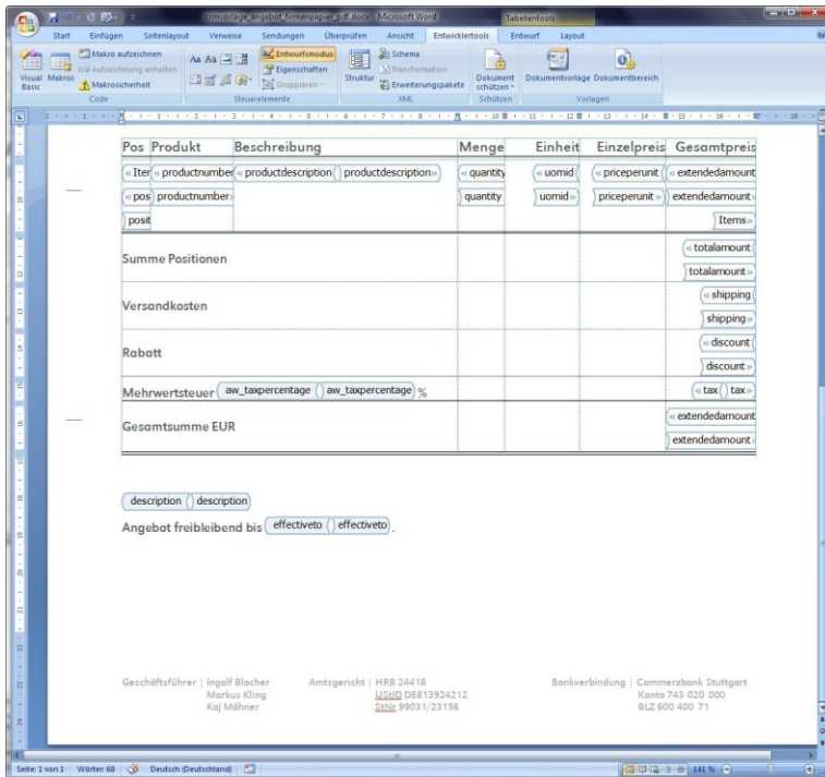
Abbildung 6 Vorlagenentwurf
