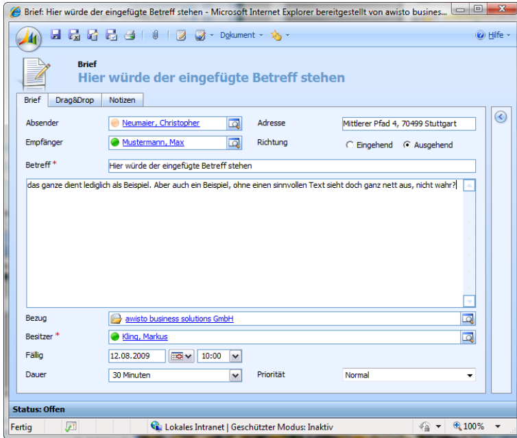
Abbildung 4 Briefaktivität
