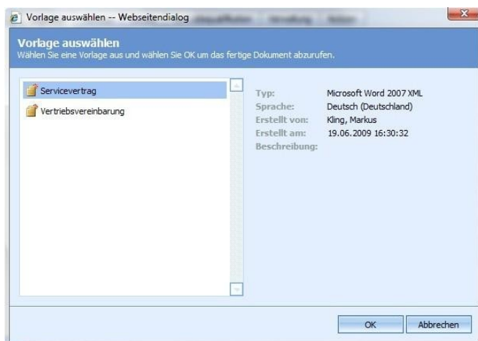
Abbildung 1 Vorlagenauswahl
