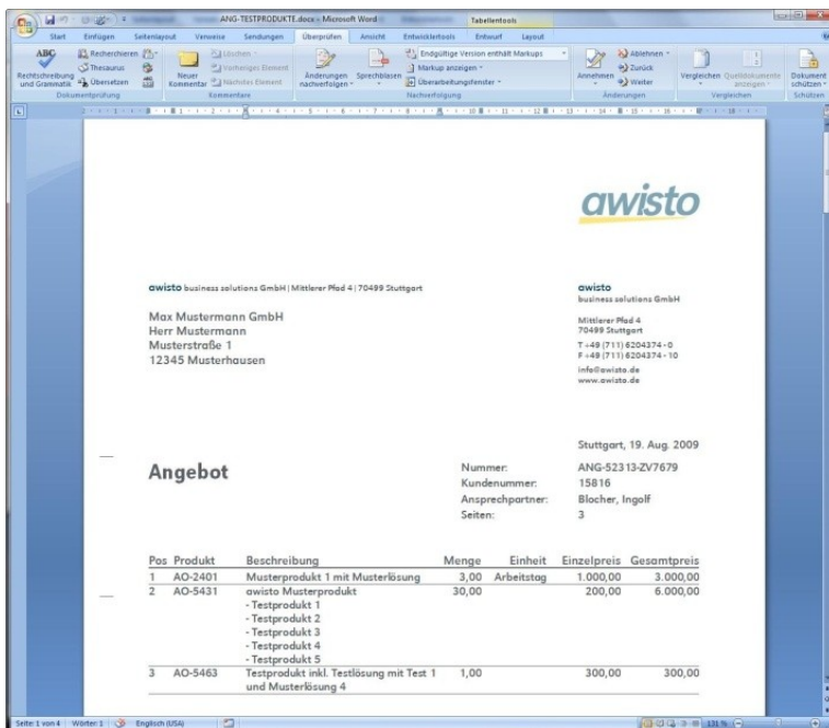
Abbildung 7 Fertiges Dokument
